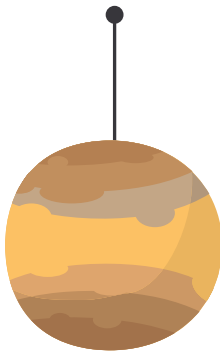
Jupiter
